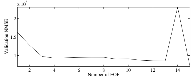
Fig. 11. EOF validation errors of the 3 rd time series using SOM grid size 8 \times 8 .
